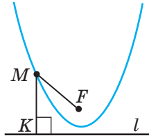
Парабола |MF| = d(M; l)
