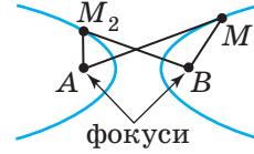
Гіпербола AM_1 - M_1B = BM_2 - M_2A = \text{const}
